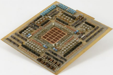
Mémoire à tores de ferrite
